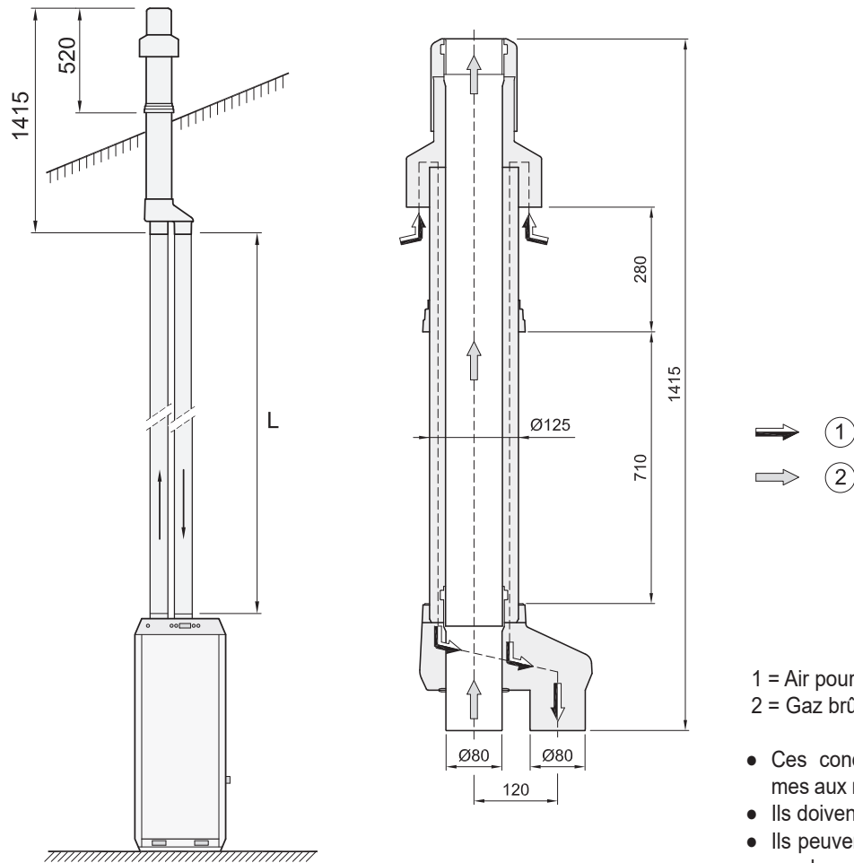
Amenée et évacuation verticales parallèles d'appareil Allure
